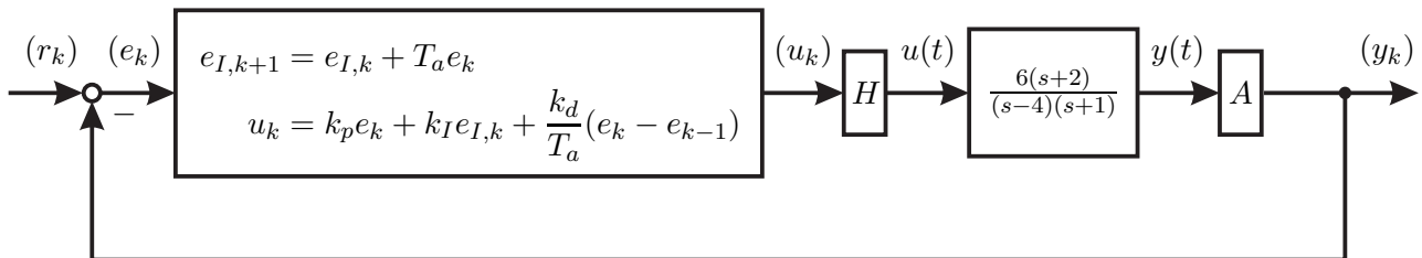
Abbildung 1: Regelkreis für die Aufgaben 23 bis 25.
