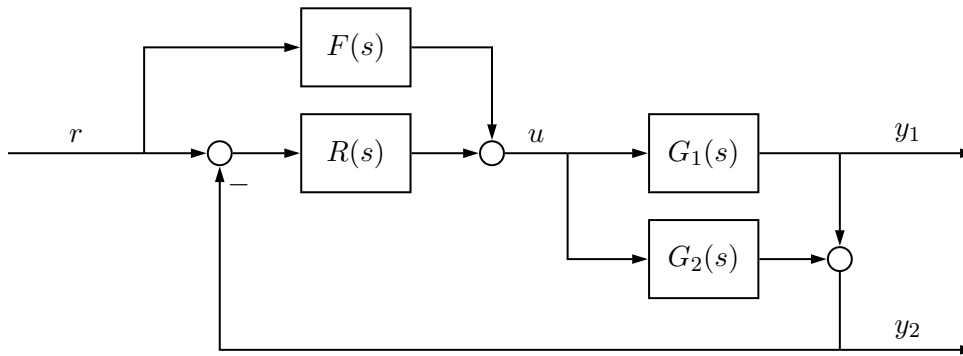
Abbildung 2: Blockdiagramm.
