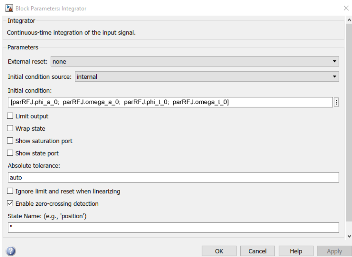
Abbildung 2.5: Berücksichtigung des Anfangszustandes \mathbf{x}_0 im Integrator-Block.
