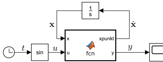
Abbildung 2.2: Implementierung von (2.12) mittels einer Matlab Function.
