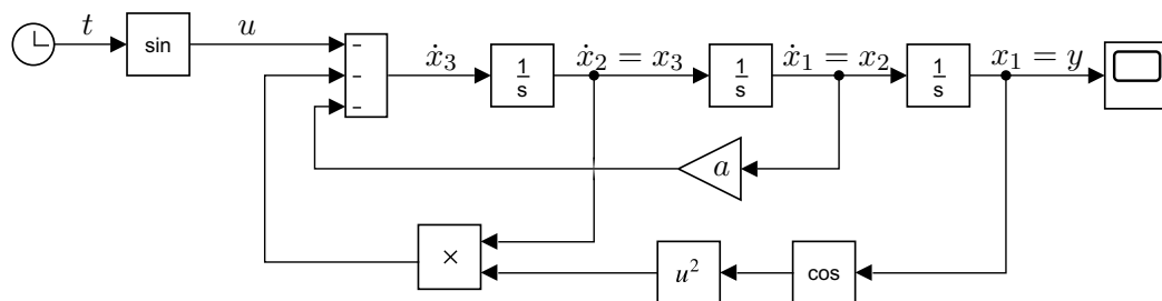
Abbildung 2.1: Implementierung von (2.12) mittels einer Integratorkette.
