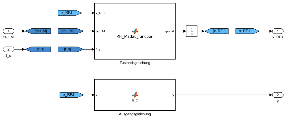
Abbildung 2.4: Struktur zur Implementierung des nichtlinearen Rotary Flexible Joint Modells in SIMULINK.
