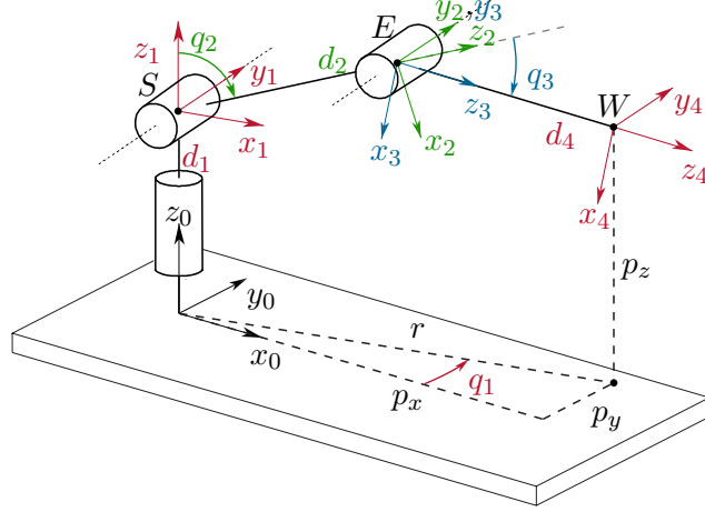
Abbildung 2.5: 3-Achs-Roboter in RRR-Struktur [2.2].
