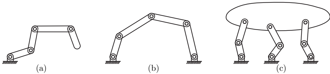
Abbildung 1.3: Kinematische Ketten [1.2]: (a) Offene bzw. serielle Kette, (b) geschlossene Kette, (c) Parallele Kinematik.
