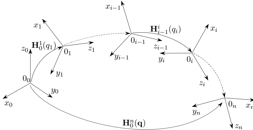
Abbildung 2.3: Koordinatensysteme eines Roboters mit serieller Kinematik [2.2].
