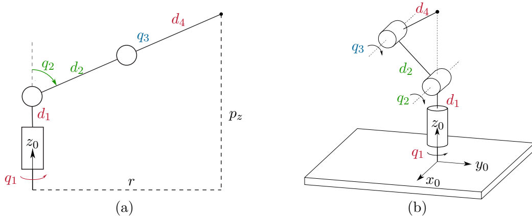
Abbildung 2.14: Kinematische Singularitäten des 3-Achs-Roboters: (a) Ausgestreckter Roboterarm ( S_1 = 0 ), (b) Endeffektor liegt auf z_0 -Achse ( S_2 = 0 ) [2.2].
