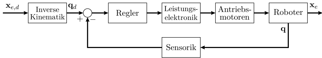
Abbildung 1.4: Regelung im Konfigurationsraum [1.1].
