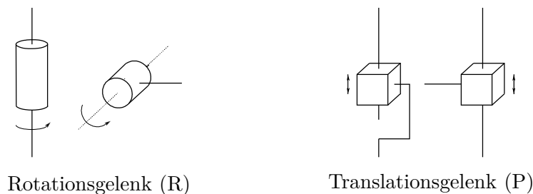
Abbildung 1.2: Schematische Darstellung eines Rotations- und eines Translationsgelenkes [1.1].
