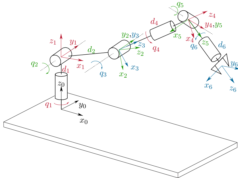
Abbildung 2.4: 6-Achs-Roboter mit sphärischem Handgelenk [2.2].
