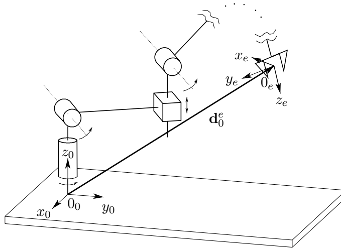
Abbildung 2.2: Schematische Darstellung einer seriellen kinematischen Kette [2.2].
