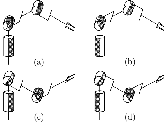
Abbildung 2.7: Vier Konfigurationen für die inverse Kinematik des 3-Achs-Roboters: (a) Shoulder-Right/Elbow-Up, (b) Shoulder-Left/Elbow-Up, (c) Shoulder-Right/Elbow-Down, (d) Shoulder-Left/Elbow-Down [2.2].
