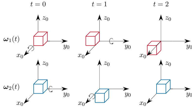
Abbildung 2.11: Bewegung des Starrkörpers, welcher mit \boldsymbol{\omega}_1(t) bzw. mit \boldsymbol{\omega}_2(t) rotiert wird [2.2].
