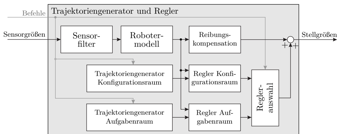
Abbildung 4.2: Blockschaltbild der Implementierung eines Trajektoriengenerators und Reglers für einen Industrieroboter.
