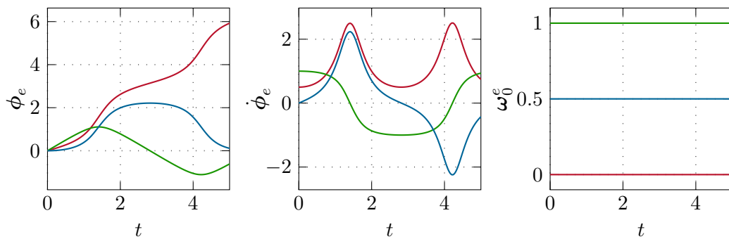
Abbildung 2.13: Drehung eines Starrkörpers mit konstantem Vektor der Drehwinkelgeschwindigkeiten \omega_e .
