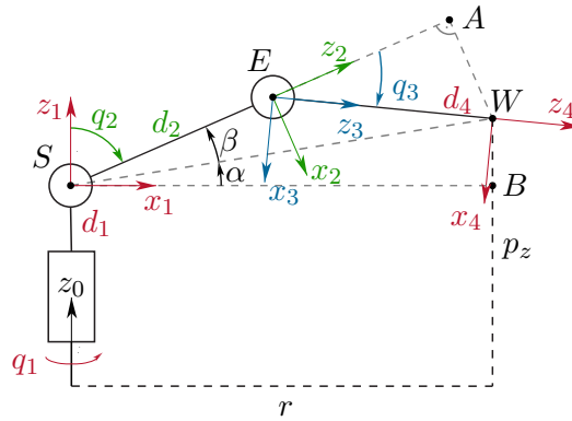
Abbildung 2.6: Ansicht der z_0 - r -Ebene des 3-Achs-Roboters.
