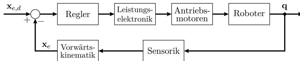
Abbildung 1.5: Regelung im Aufgabenraum, angepasst von [1.1].
