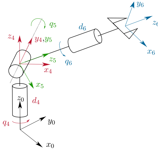
Abbildung 2.8: Sphärisches Handgelenk [2.2].
