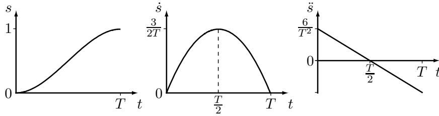
Abbildung 3.2: Schematische Darstellung der Funktionen s(t) , \dot{s}(t) und \ddot{s}(t) für die Zeitparametrierung mithilfe eines Polynoms 3. Ordnung [3.1].
