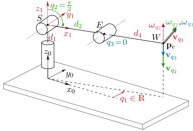
Abbildung 2.10: Translatorische Geschwindigkeiten \mathbf{v}_{q_i} und Drehwinkelgeschwindigkeiten \boldsymbol{\omega}_{q_i} am Endeffektor des 3-Achs-Roboters in der Konfiguration \tilde{\mathbf{q}} = [q_1 \ \frac{\pi}{2} \ 0] zufolge der Gelenksgeschwindigkeiten \dot{q}_i = 1 , i = 1, 2, 3 .
