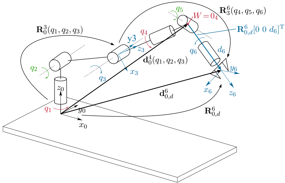
Abbildung 2.9: Inverse Kinematik des 6-Achs-Roboter mit sphärischem Handgelenk [2.2].
