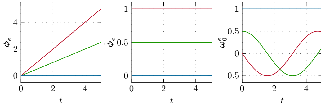
Abbildung 2.12: Drehung eines Starrkörpers mit konstanter Drehrate \dot{\phi}_e in Minimalkoordinatendarstellung mit RPY-Winkel.
