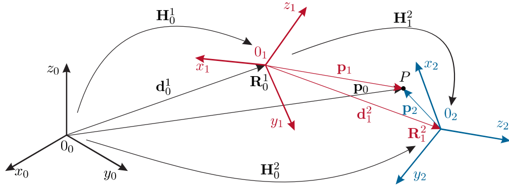
Abbildung 2.1: Homogene Transformationen am Beispiel der Koordinatensysteme (0_0 x_0 y_0 z_0) , (0_1 x_1 y_1 z_1) und (0_2 x_2 y_2 z_2) [2.1].
