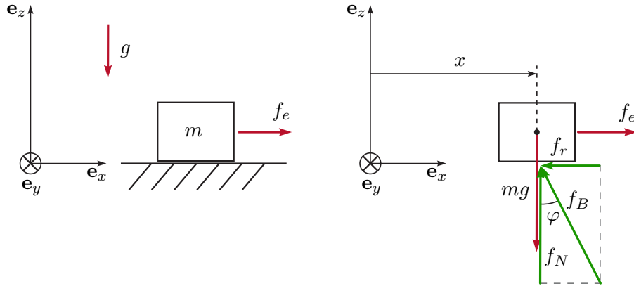
Abbildung 3.22: Zur Haftreibung.
