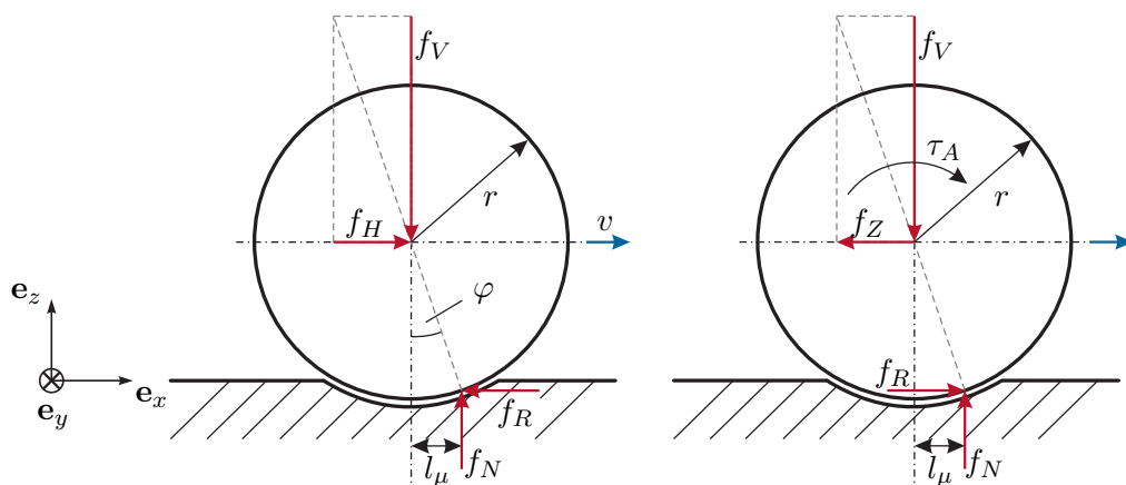
Abbildung 3.28: Lauf- und Treibrad.
