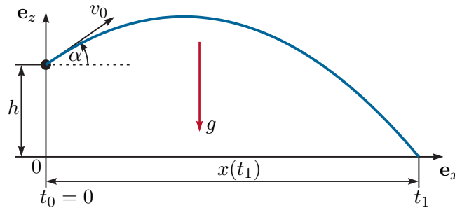
Abbildung 3.15: Wurfparabel.
