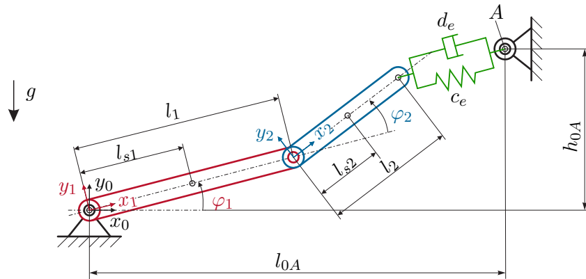
Abbildung 5.9: Skizze des planaren Manipulators.
