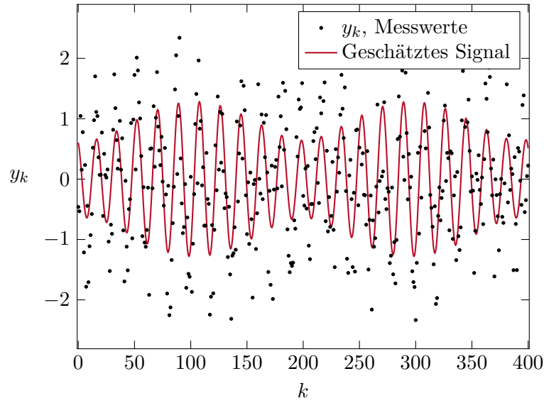
Abbildung 3.4: Messwerte und geschätzter Verlauf des unverrauschten Signals.
