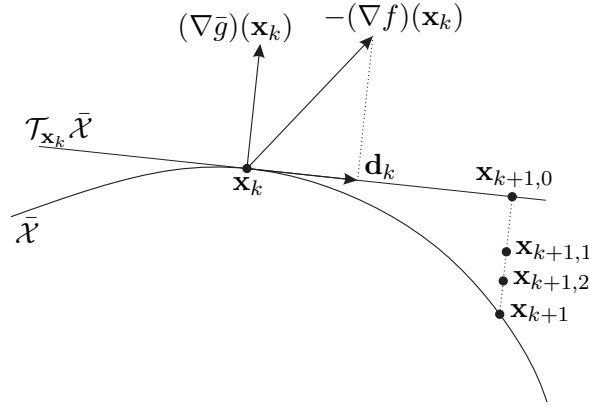
Abbildung 3.5: Gradienten-Projektionsmethode.
