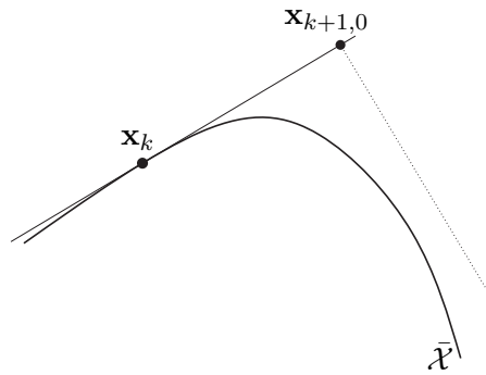
Abbildung 3.6: Nichtexistenz von \boldsymbol{\eta}_k , um auf \bar{\mathcal{X}} zu kommen.
