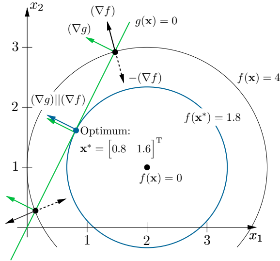
Abbildung 3.2: Veranschaulichung von Beispiel 3.3 mit einer Gleichungsbeschränkung.
