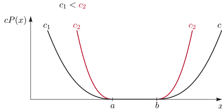
Abbildung 3.8: Strafffunktionen cP(x) für verschiedene Werte von c .
