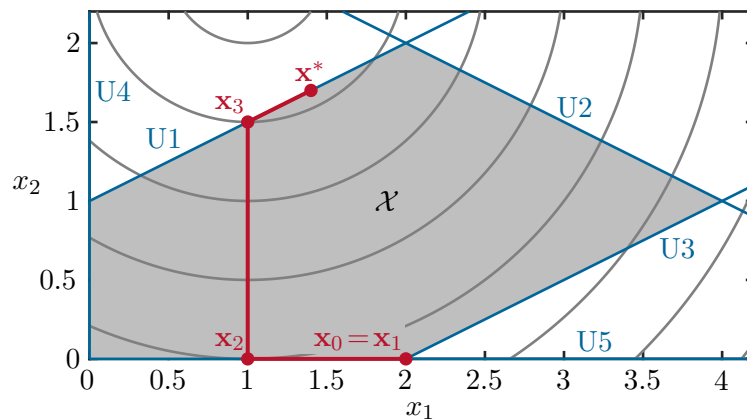
Abbildung 3.4: Anwendung der Methode der aktiven Beschränkungen auf das beschränkte quadratische Optimierungsproblem (3.87).
