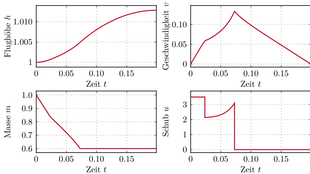
Abbildung 1.8: Trajektorien für die Goddard-Rakete.
