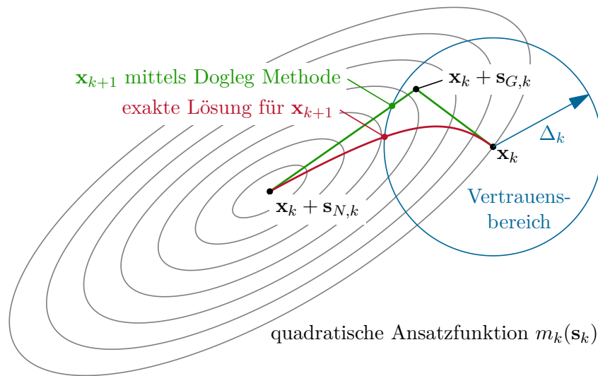
Abbildung 2.8: Lösung des Optimierungsproblems (2.115) im Rahmen einer Iteration der Methode der Vertrauensbereiche, Vergleich zwischen exakter Lösung (rot) und Dogleg Methode (grün).
