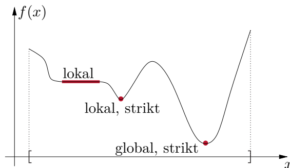
Abbildung 1.10: Verschiedene Minima einer Funktion f(x) mit x \in \mathbb{R} .
