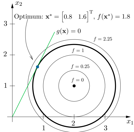
Abb. 1.3: Geometrische Darstellung des beschränkten Optimierungsproblems (1.10), (1.11).
