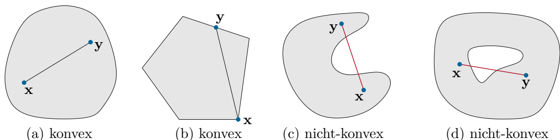
Abbildung 1.13: Beispiele von konvexen und nicht-konvexen Mengen.
