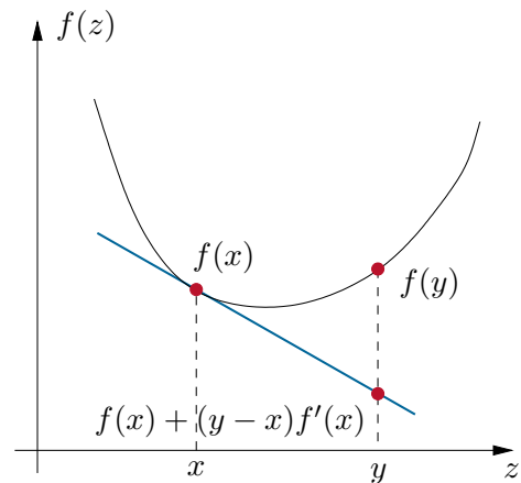
Abb. 1.16: Stützende Tangente einer konvexen Funktion f(z) .
